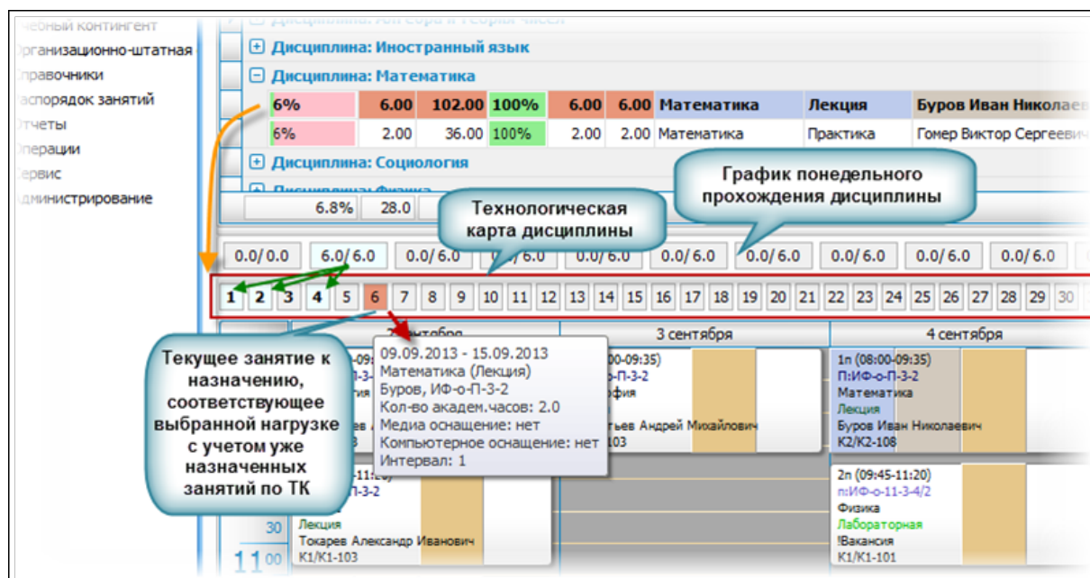
Рис. 59. Технологическая карта в конструкторе расписания
