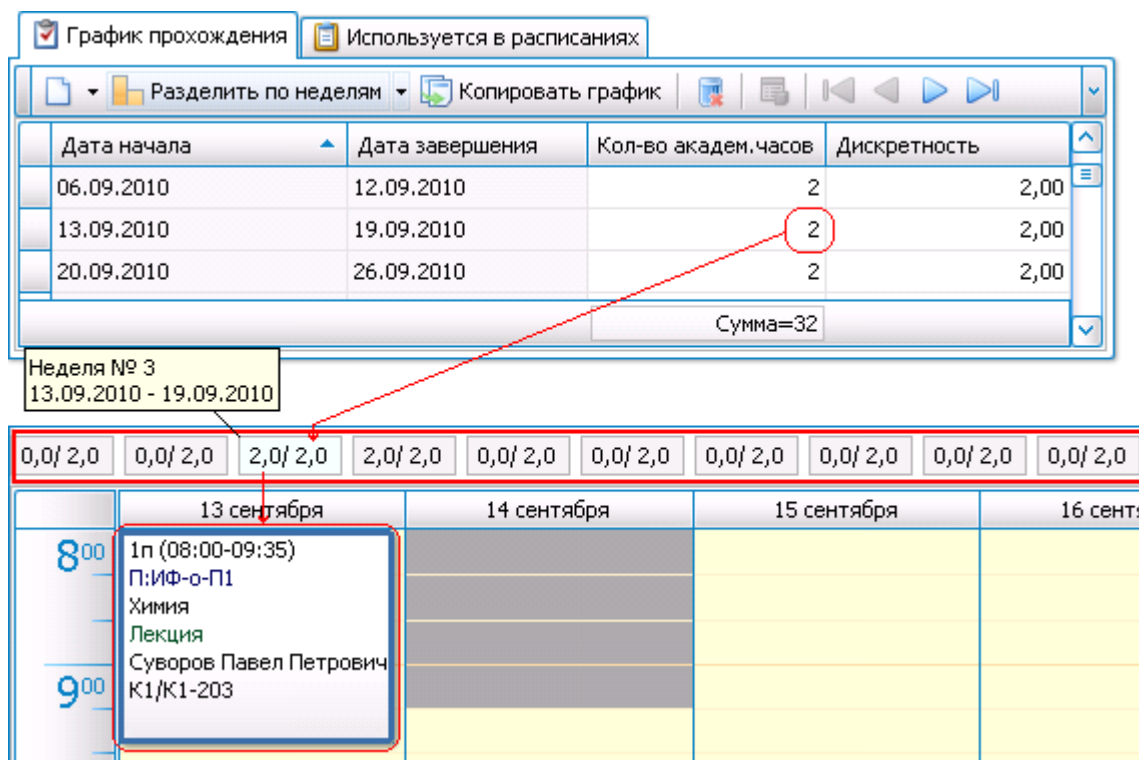
Рис. 58. График прохождения нагрузки
